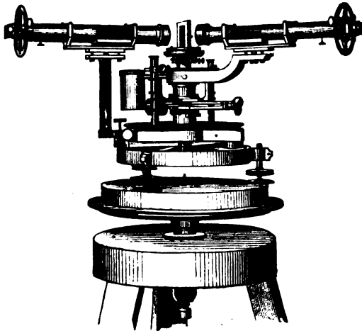
FIG. 34.—Ångström's spectrometer.
